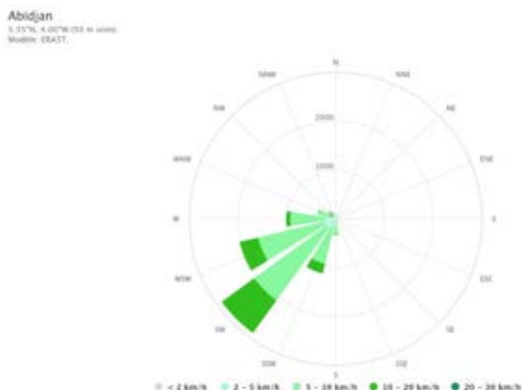
Figure 12: Directions dominantes des vents (rose des vents Abidjan) (Source : Météo Blue, 2024)
