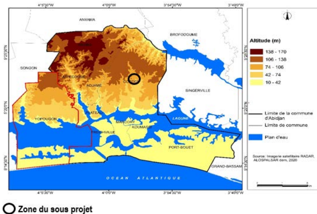
Figure 5 : Relief de la ville d'Abidjan.
