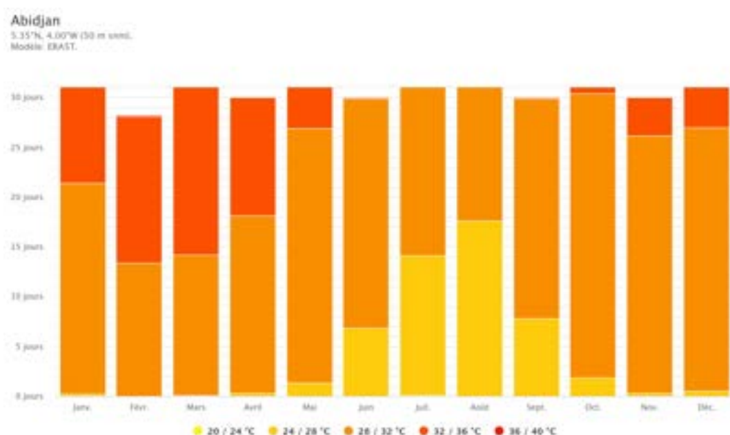
Figure 10: Températures maximales d'Abidjan, source : Météo Blue 2024
