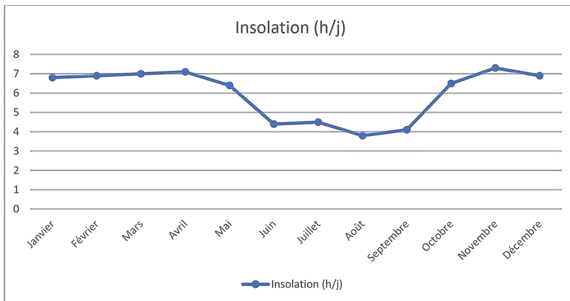
Figure 11: Courbe d'évolution de l'insolation moyenne mensuelle (2005-2020)
