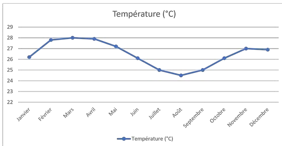
Figure 9: Courbe d'évolution de la température moyenne mensuelle (1995-2020)
