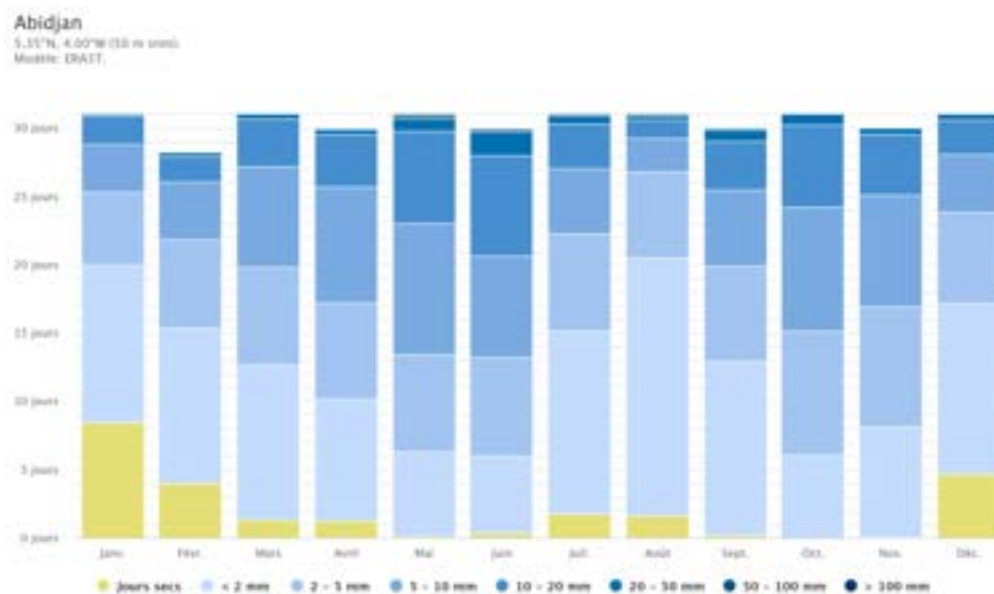
Figure 8 : quantité de précipitations Abidjan, source : Météo Blue 2024
