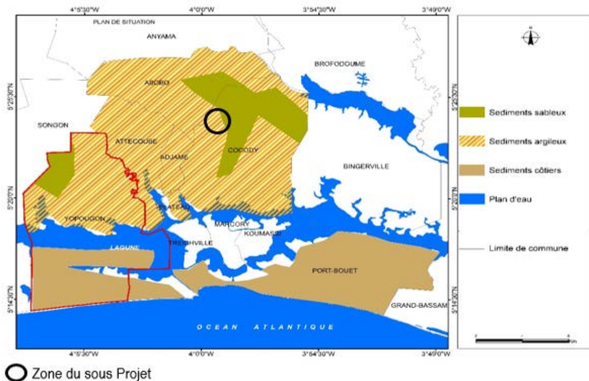
Figure 6 : Contexte géologique de la ville d'Abidjan (source : NEXON Consulting, 2023)
